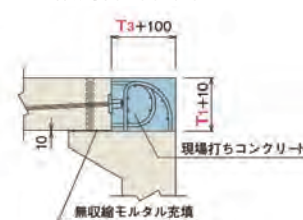
隅角部詳細図
