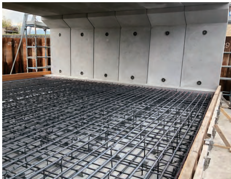
底版配筋状況
