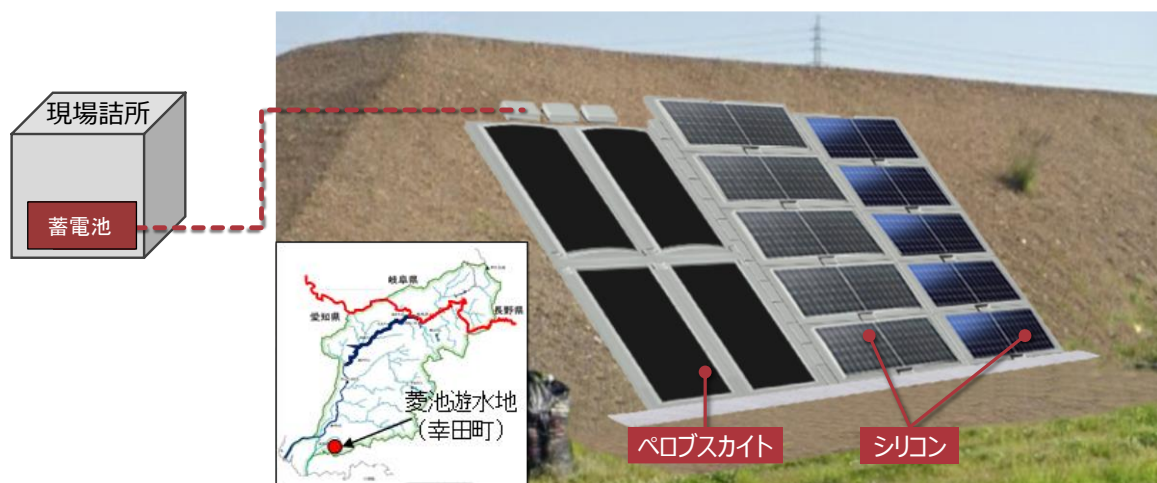
太陽光発電システム設置イメージ図
